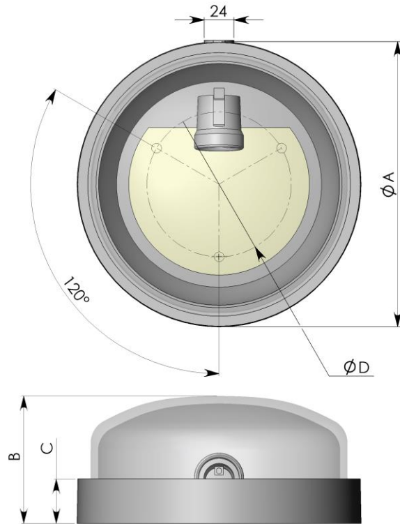
Рис. 2. Габаритні та монтажні розміри світильника
